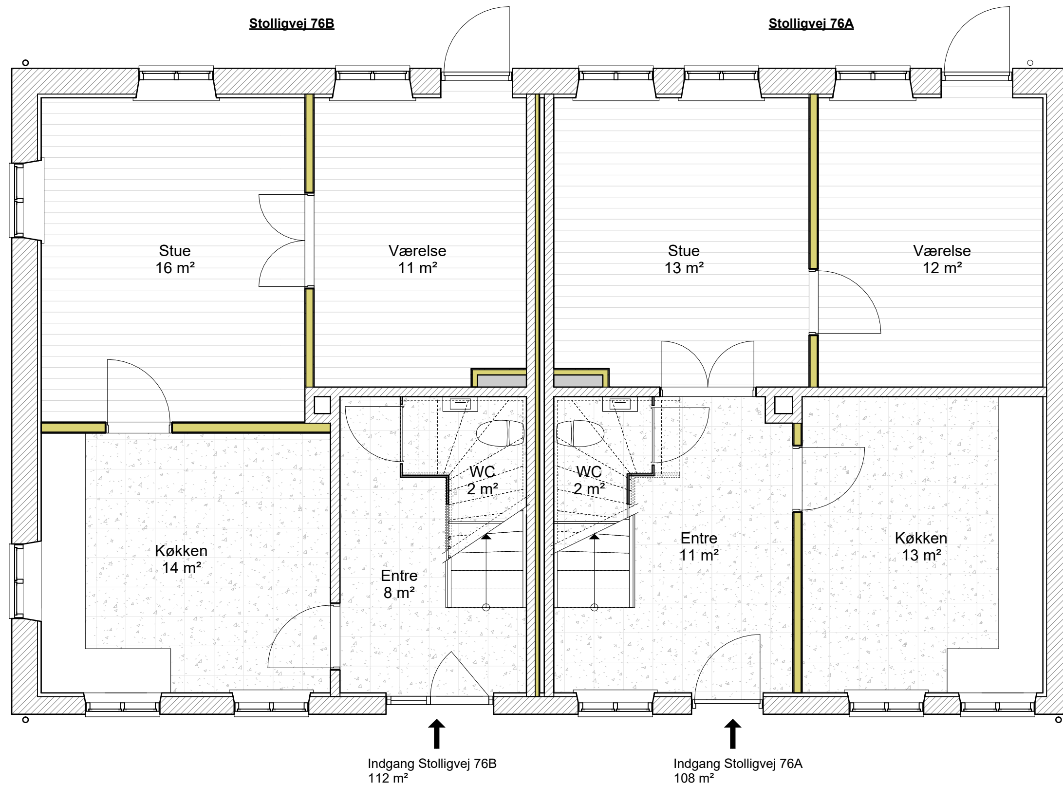
Stueplan 1 : 50
